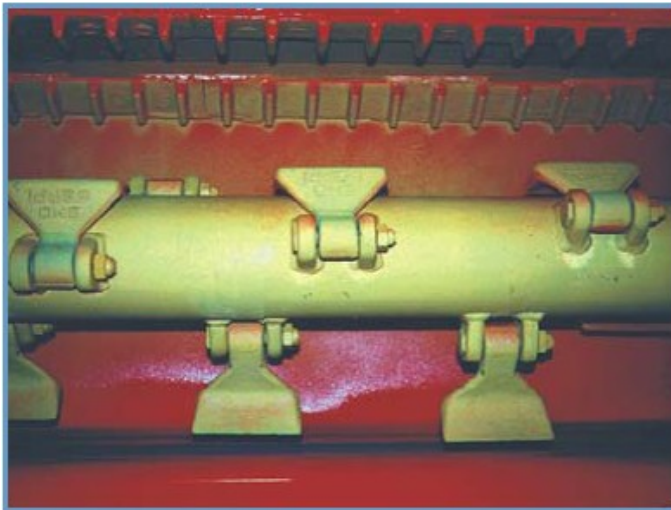
Rotor cu ciocane montate in spirala si contracutit forjat. Dotare standard pentru SMWA-avs si SMO-avs
