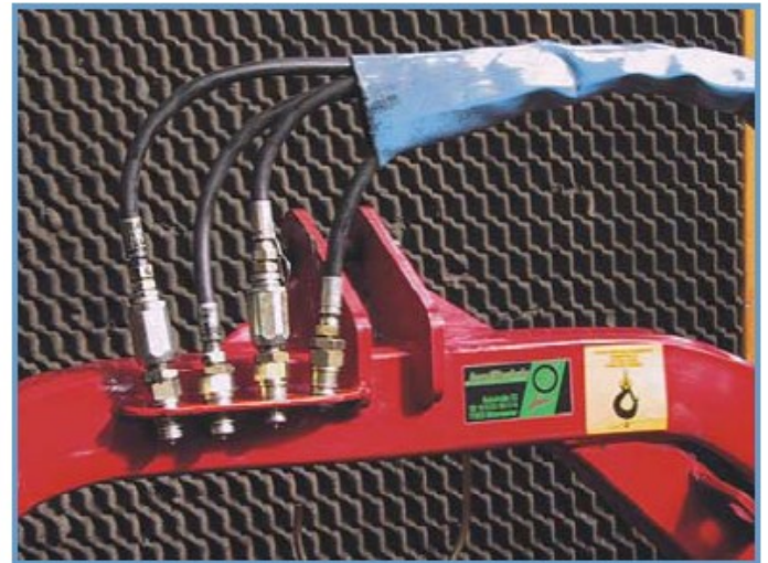
Suport de sustinere a elementelor de cuplaj rapid
